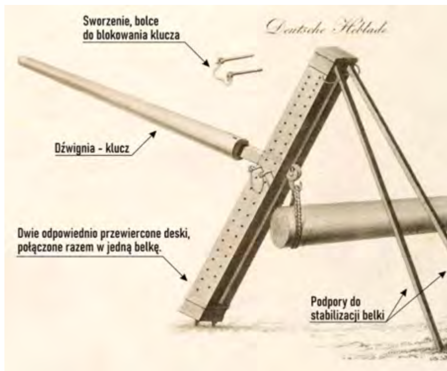
Fragment ilustracji technicznej dostosowanej na potrzeby artykułu zawierającej szkic „Deutsche Hebelade”, ok 1890 r.
